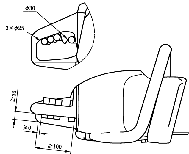
图 2 后手把防护的最小尺寸
