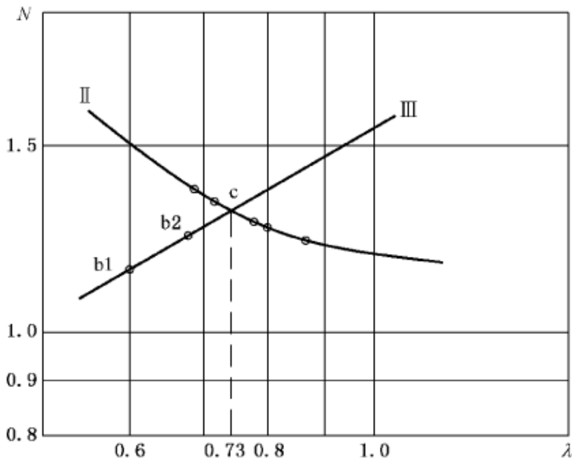
图 B.2 修正气水比计算图
