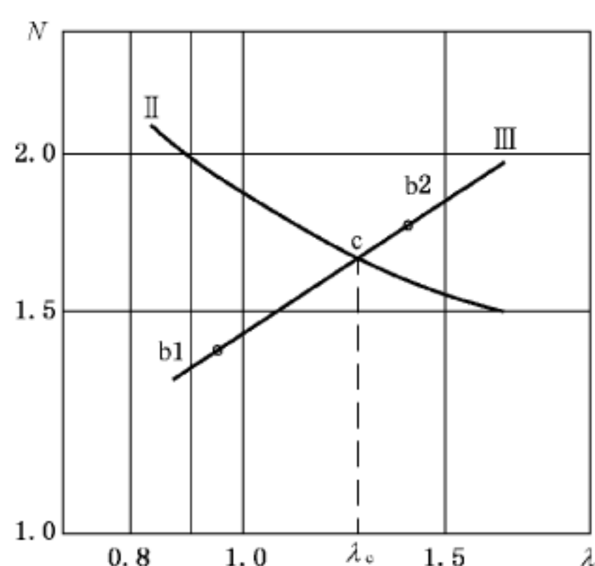
图 A.2 修正气水比计算图
