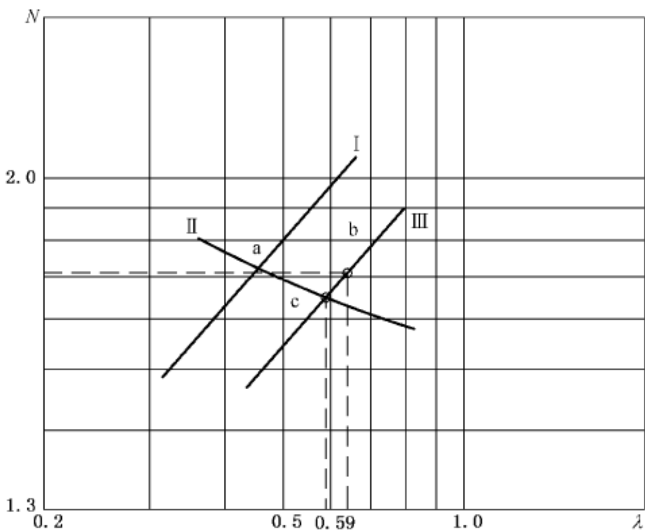
图 B.1 修正气水比计算图
