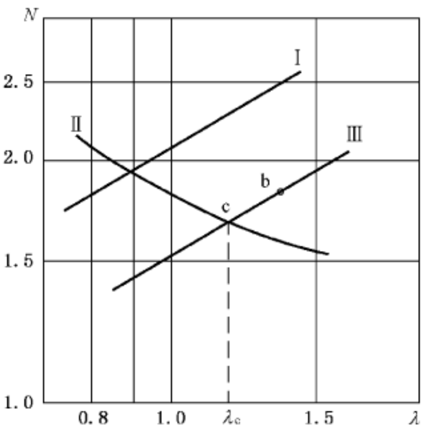
图 A.1 修正气水比计算图
