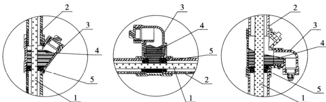
图 B.0.4 隔离密封盒安装示意图
