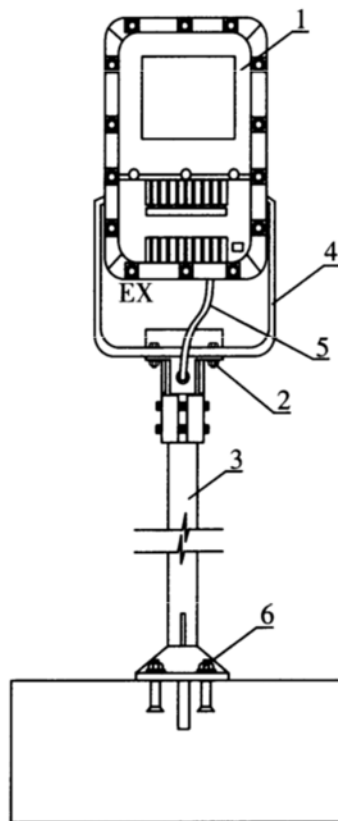
图 B.0.7-3 投光灯立柱式安装示意图
