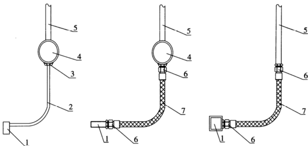
图 B.0.9 防爆仪表安装示意图
