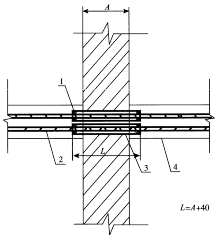
图 B.0.6 金属桥架穿墙的隔离封堵示意图
