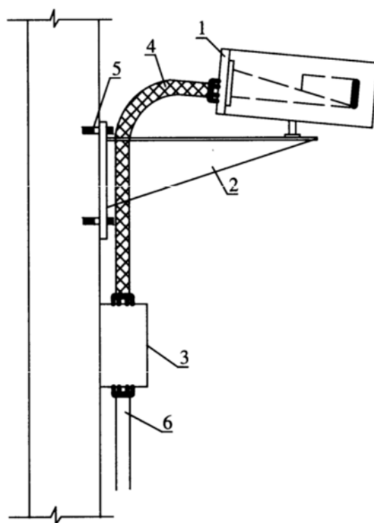
图 B. 0. 10 防爆摄像机壁式安装示意图 1—防爆摄像机；2—安装支架；3—防爆接线箱； 4—防爆挠性管；5—膨胀螺栓；6—钢管
