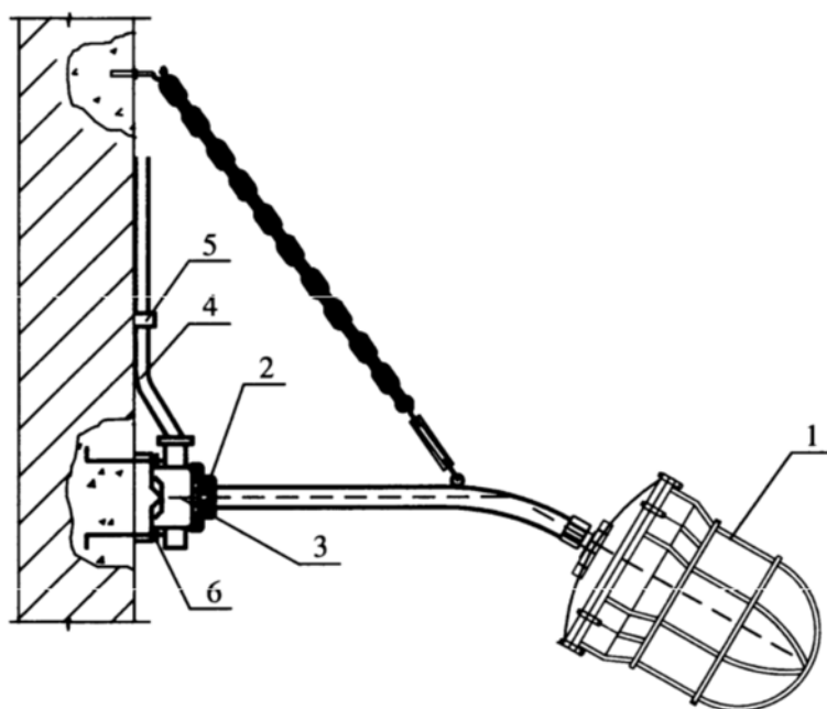
图 B.0.8-3 防爆灯壁式安装示意图
