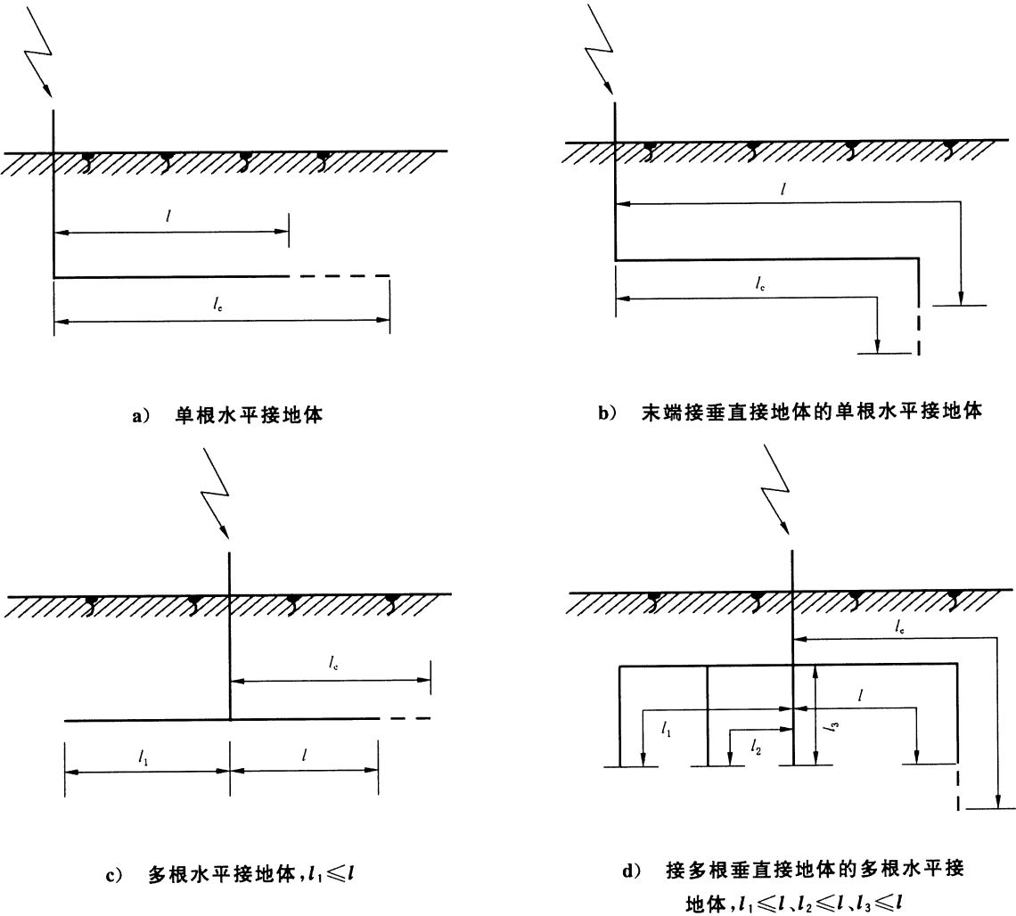
图 H.2 接地体的有效长度
