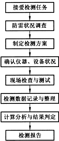
图 1 防雷装置检测工作程序框图
