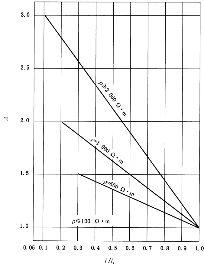
图 H.1 换算系数 A
