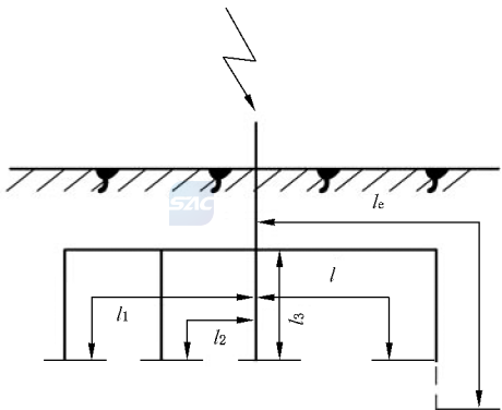
d) 接地根垂直接地的多根水平接地体, l_1 \leq l 、 l_2 \leq l 、 l_3 \leq l
