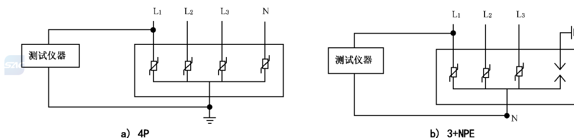
图 1 SPD 测试示意图
