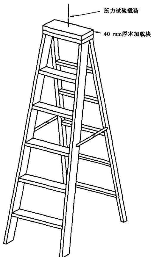
图5 压力试验加载示意图
