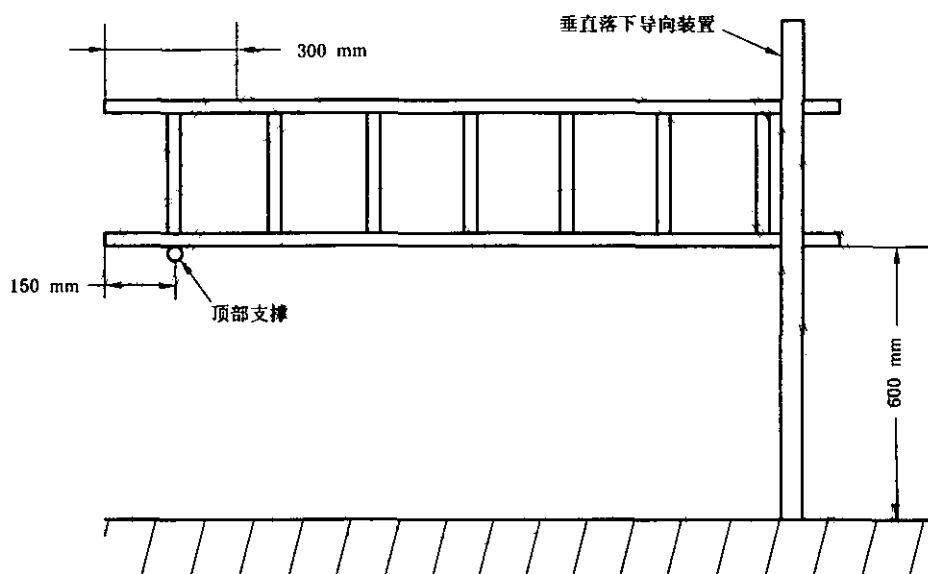
图 2 梯框悬臂落下试验示意图
